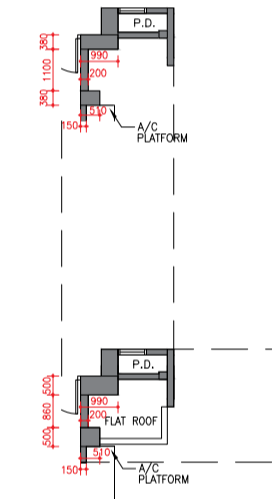
28/F PART PLAN 28樓之部分平面圖
